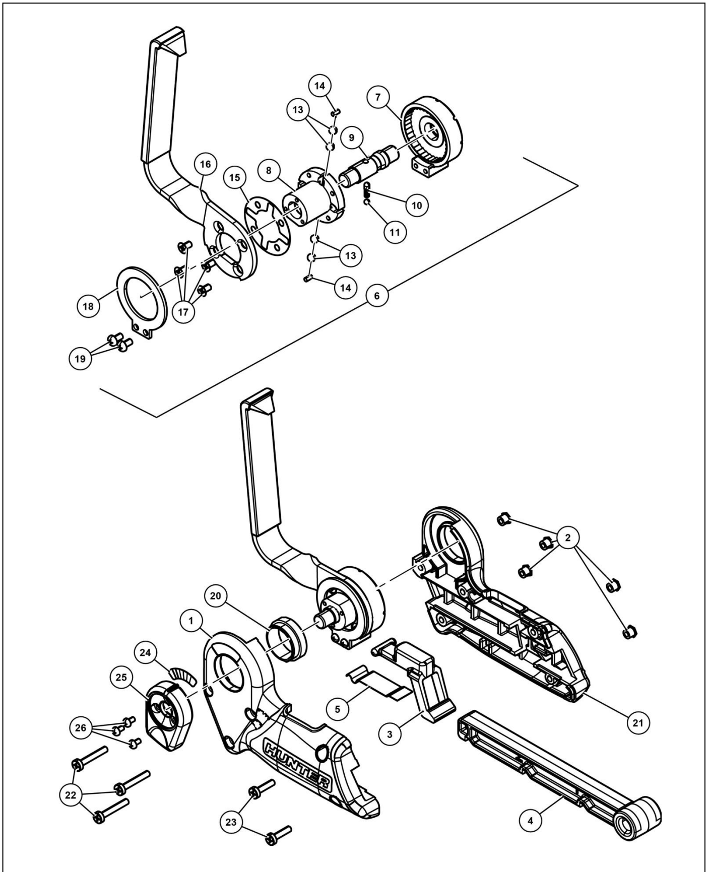
ADJUSTABLE TIRE HOOK - 142-163-1 / 142-164-1
